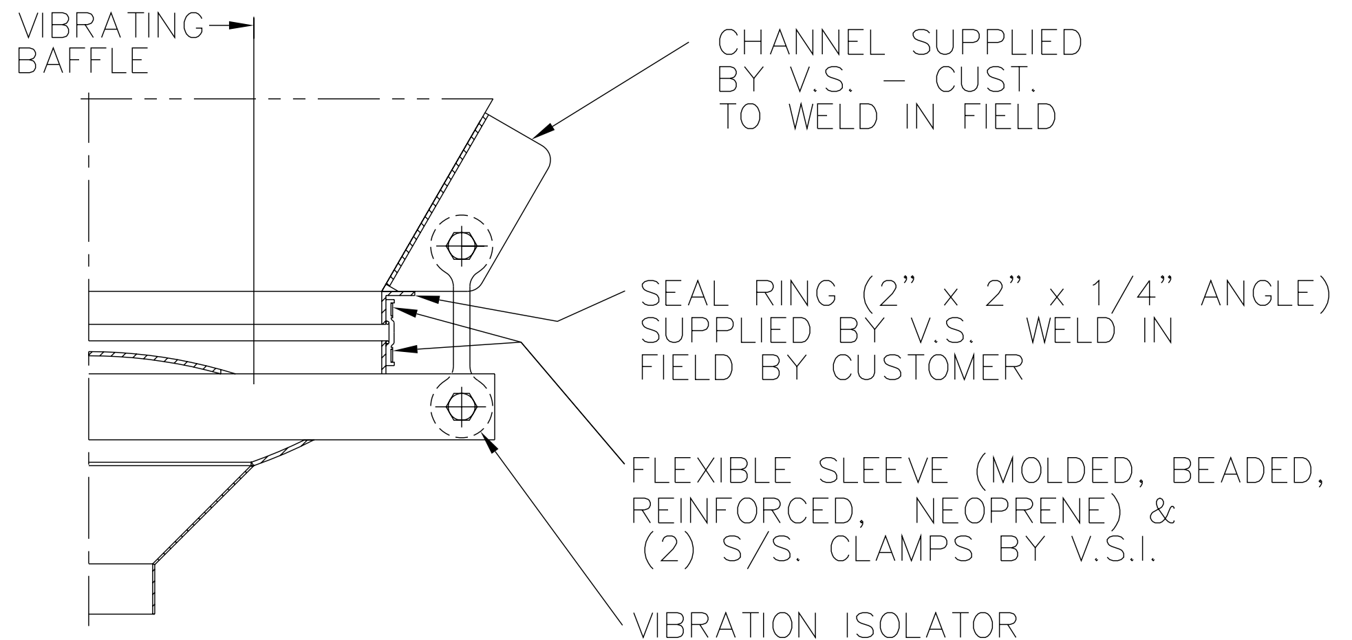
SECTION A-A
