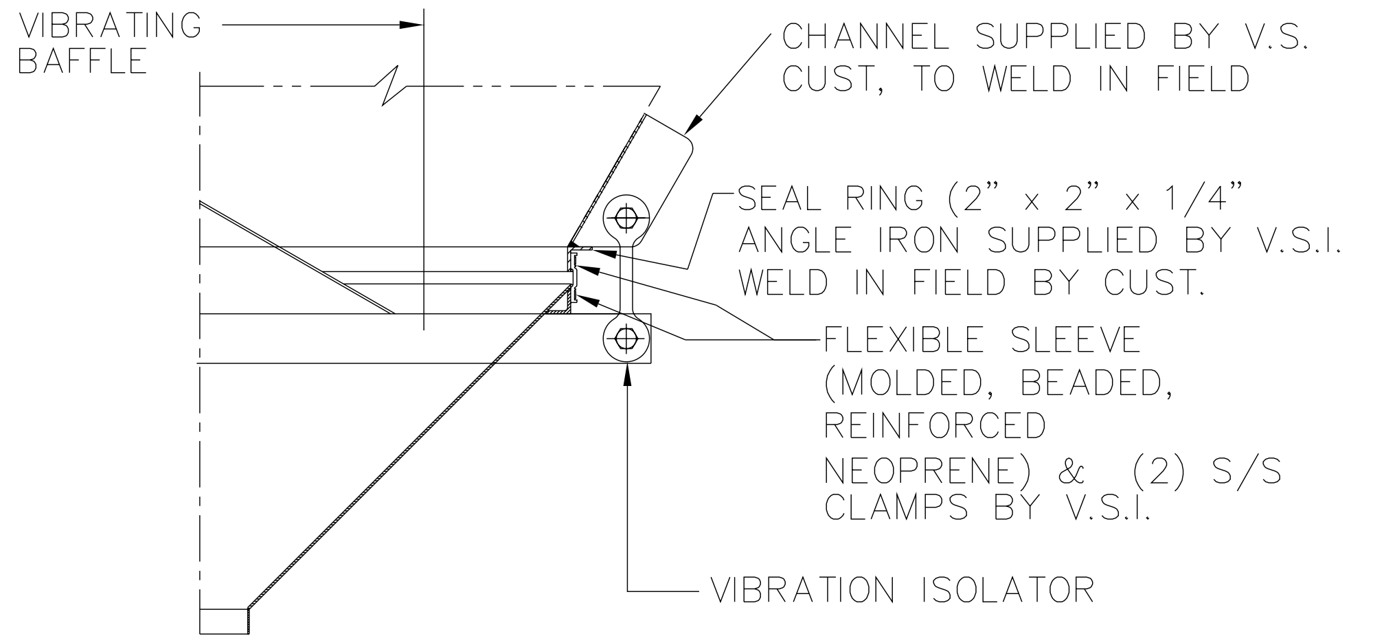
SECTION A-A
