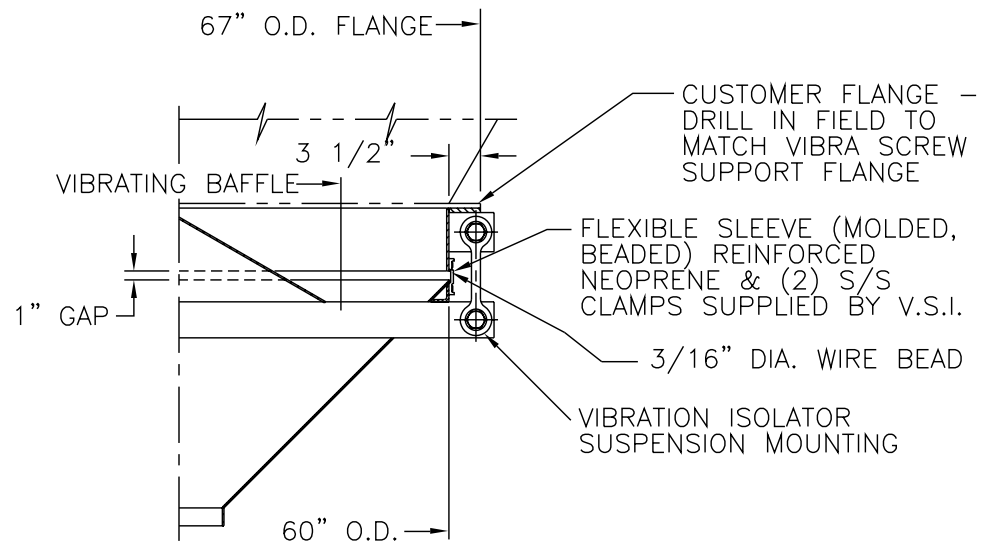
SECTION A-A
